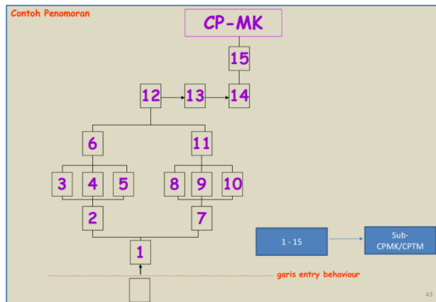
Gambar 3.2 Diagram hasil analisis pembelajaran mata kuliah Matematika Teknik
